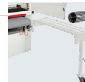
"HPL" Hobelwelle: maximaler Abtrag mit einem einzigen Arbeitsgang.
