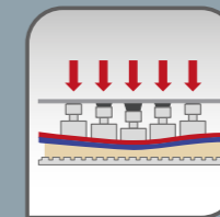
elastischer Gliederschleifschuh
