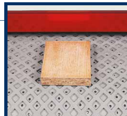
Vorschubteppich mit einem besonderen Gummiprofil in Rhombusform: bessere Übertragung der Vorschubkraft auf das Werkstück und optimale Führungsstabilität.
