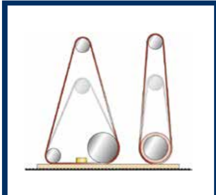
Lange Schleifbänder: 2620 mm für eine Produktivitätssteigerung verbunden mit weniger Maschinenstillständen.
