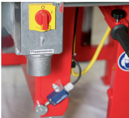
Kombi-Elektroschalter mit Phasenwender / automatische Abschaltung bei Öffnen der Haube
