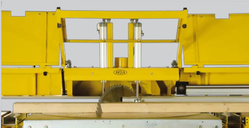
Pneumatische, verstellbare Spannzylinder
