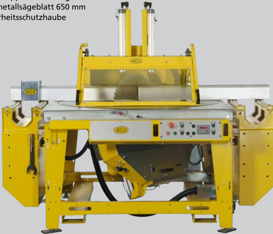
GAMA 65 K – Rollenaufgabe-/Entnahmetisch, Alu-Anschläge, Klappanschlag, horizontale Spannzylinder
